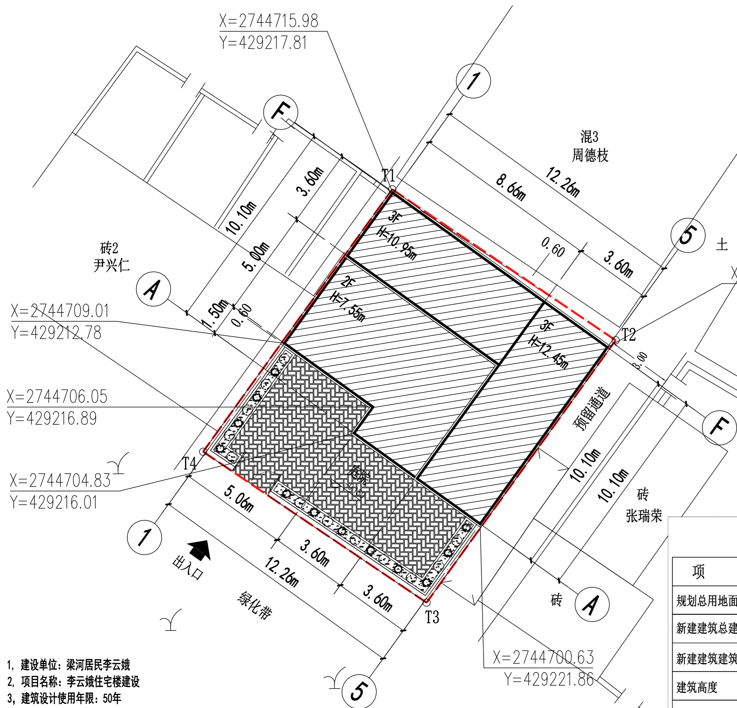
总平面布置图 1:200
